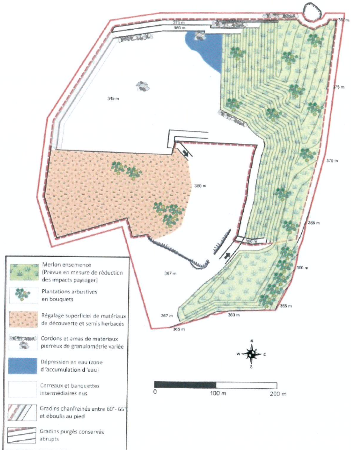
Figure 51 : Principe de la remise en état
