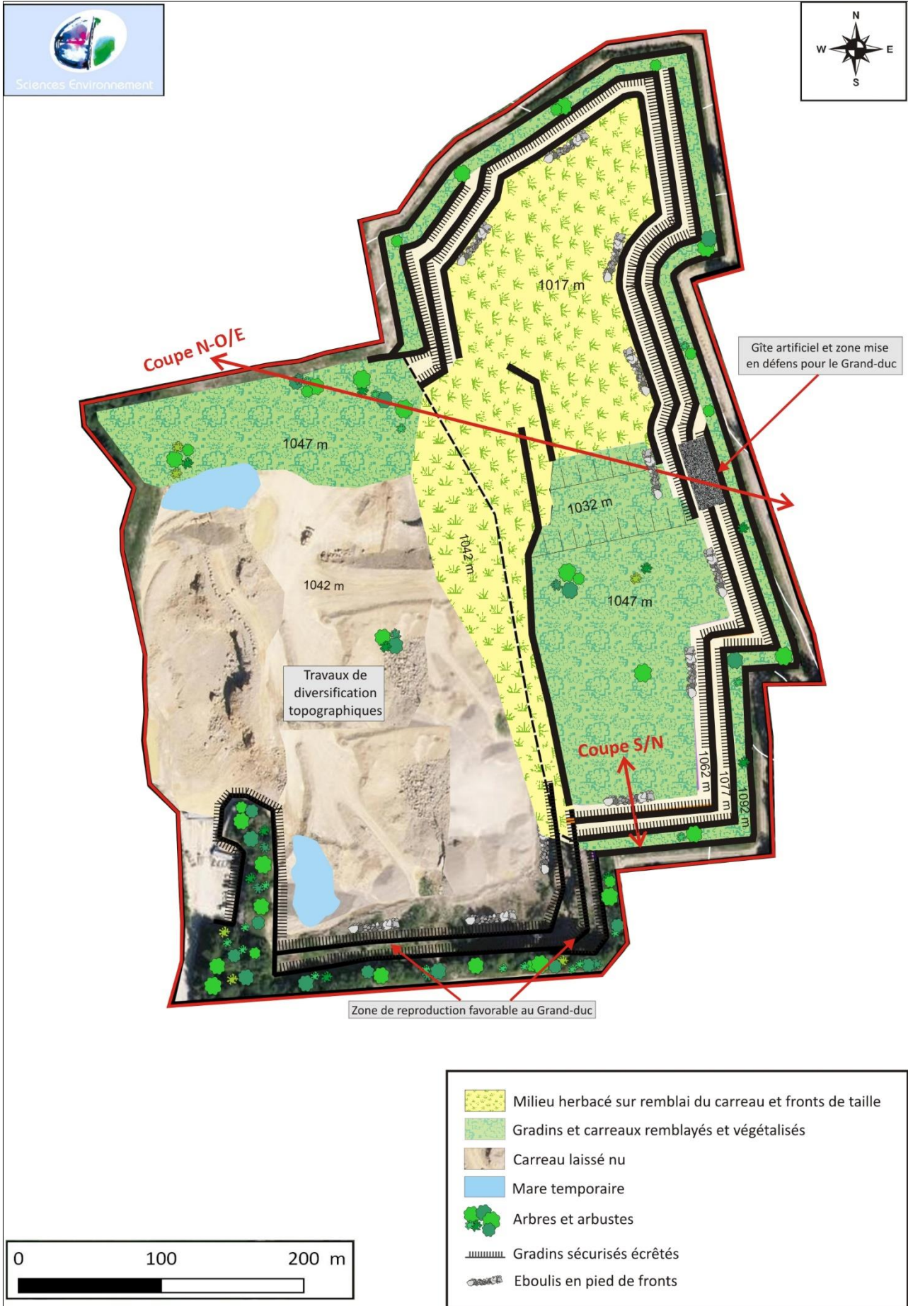
Figure 1 : Schéma de principe de la remise en état du site
